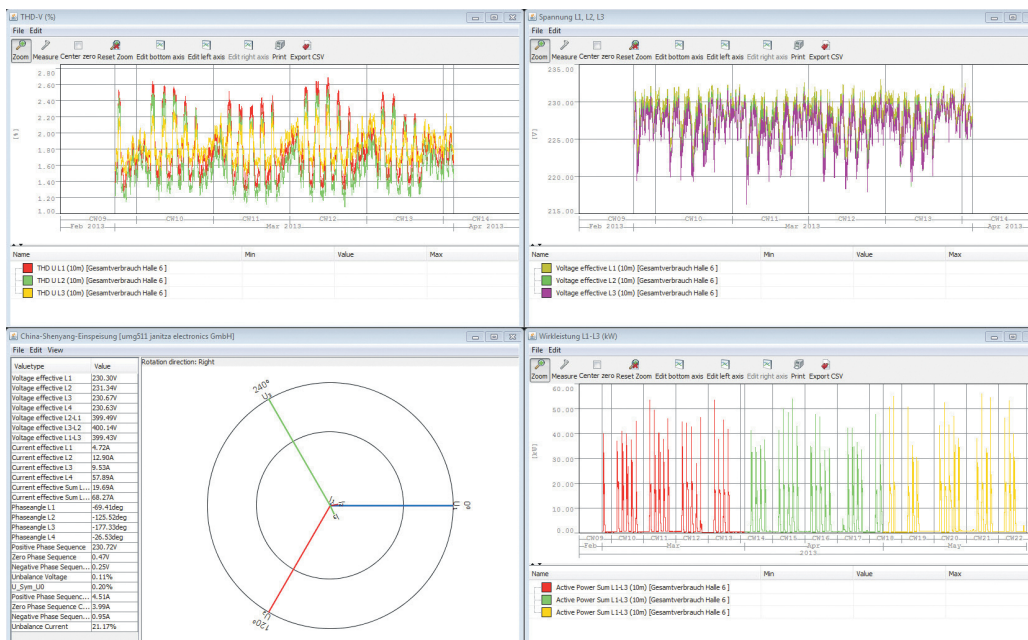
Abb.: GridVis® Graphset mit THD-U, Spannung, Zeigerdiagramm und Lastprofil
