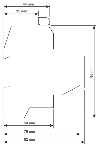
Seitenansicht
