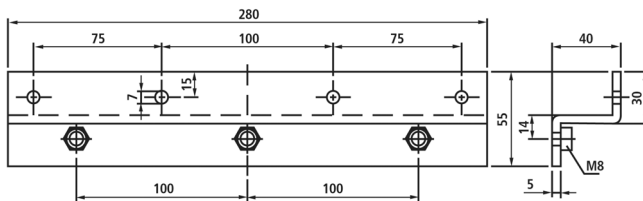
Halter Z100
