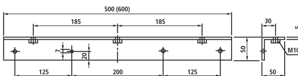
Halter L185/1
