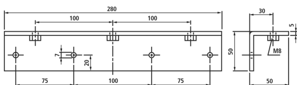
Halter L100
