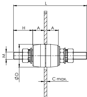
Durchgangs-Isolator Typ PI/P Polyestermaterial, rot
