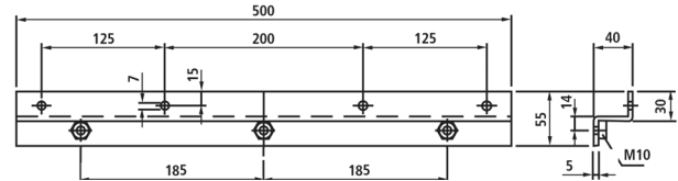
Halter Z185/1
