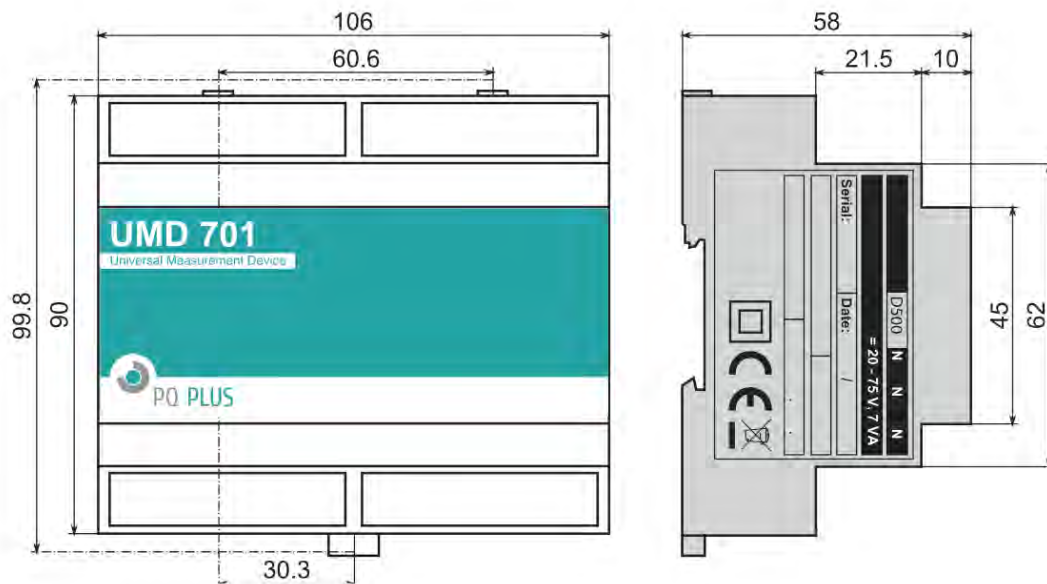
Bild 1: Abmessungen des UMD 701 Analysegeräts.
