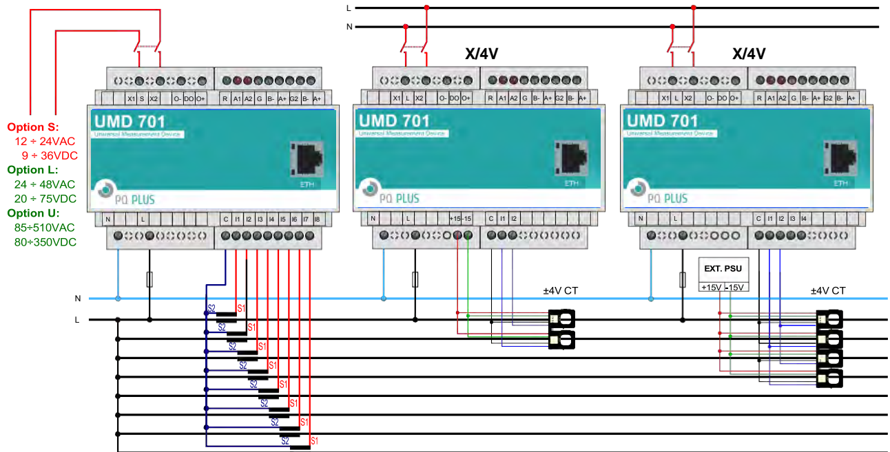
Bild 3: Beispiel einer typischen Installation des UMD 701 in einem Niederspannungsnetz — von links nach rechts: mit niedriger Versorgungsspannung (möglich: Gleichstrom, Wechselstrom auch mit Setups, abgesichert durch batteriegestützte unterbrechungsfreie Stromversorgung (USV)), versorgt aus dem gemessenen Netzwerk. Option E für Übertragung per Ethernet-Port. Option U für lokalen USB-Anschluss (alle Geräte unterstützen serielle RS485-Schnittstellen).
