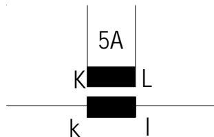
Bild 1 Anschlussbedingungen Stromwandler
